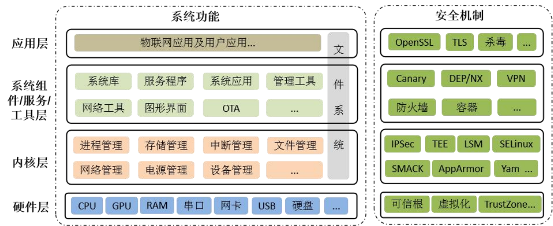
图 3 典型资源丰富型物联网操作系统及安全架构
