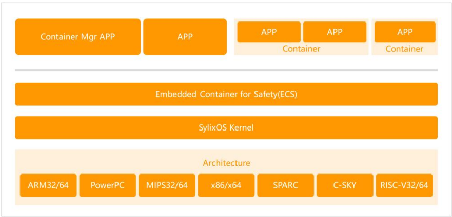
图 7 工业安全容器架构
