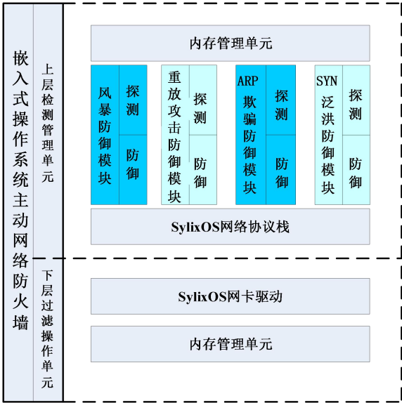
图 9 嵌入式防火墙结构图
