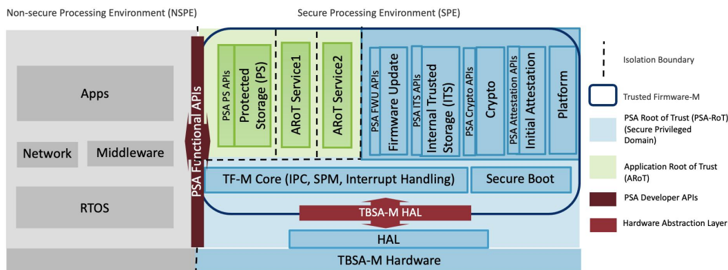
图 8 运行 TF-M 的典型系统模块框图
