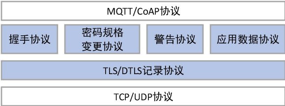
图 10 OneTLS 分层结构图
