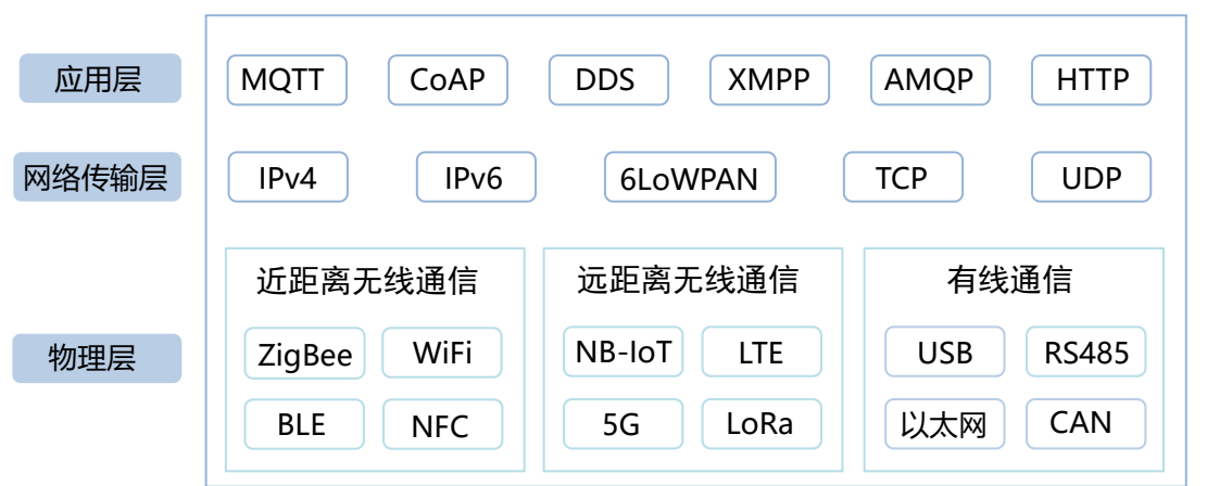
图 4 常见物联网通信协议
