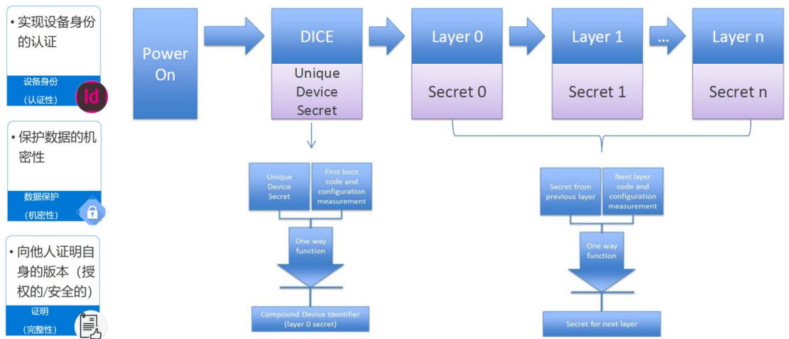
图 5 DICE-设备标识组合引擎
