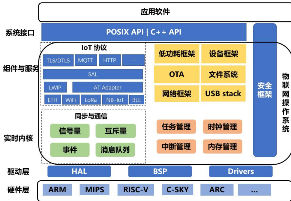
图 1 物联网操作系统架构示意图
