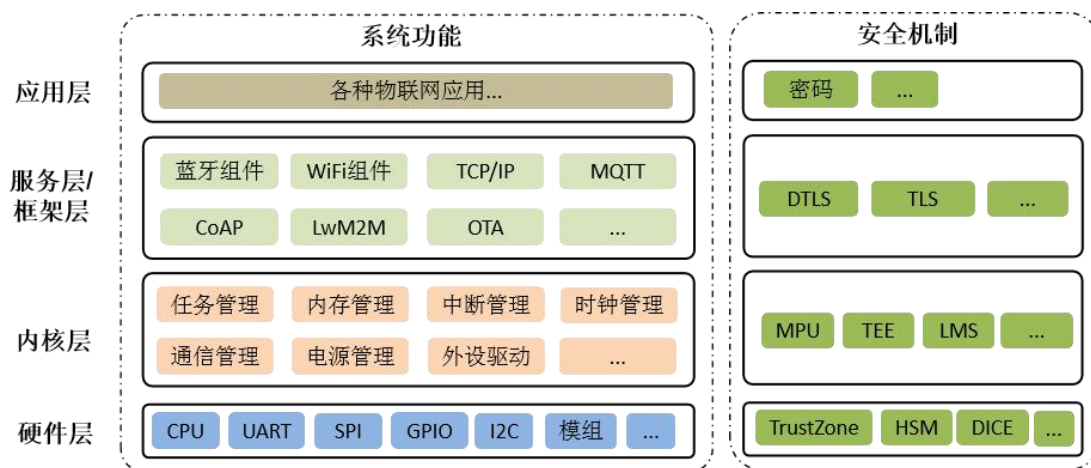
图 2 典型资源受限型物联网操作系统及安全架构
